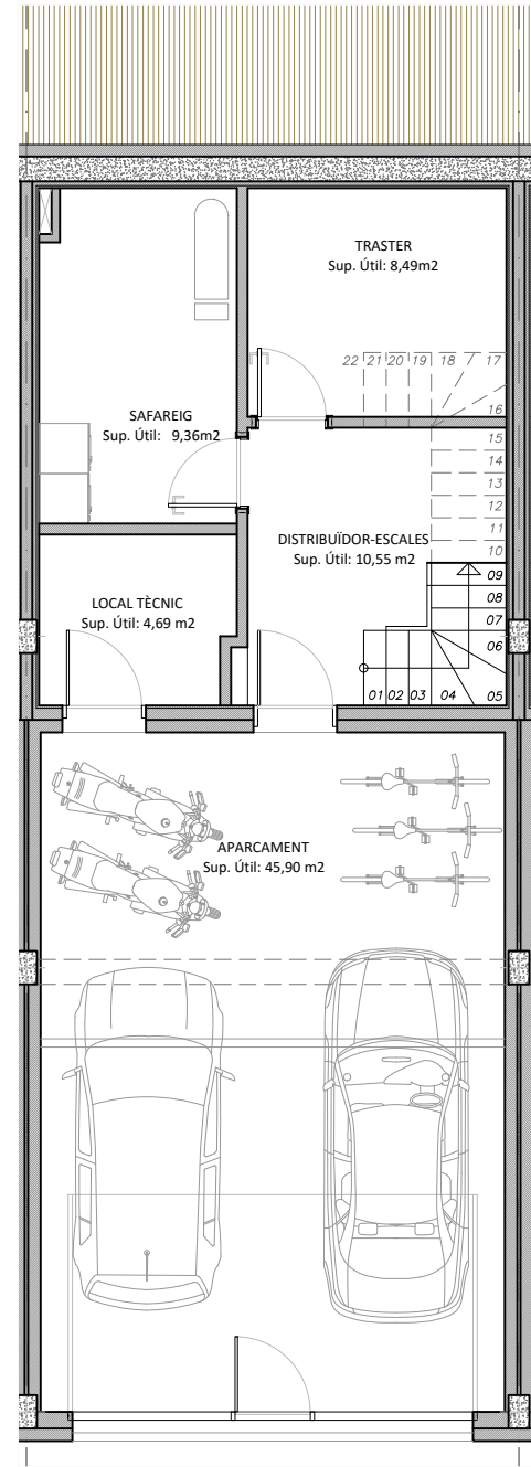
PLANTA SOTERRANI
