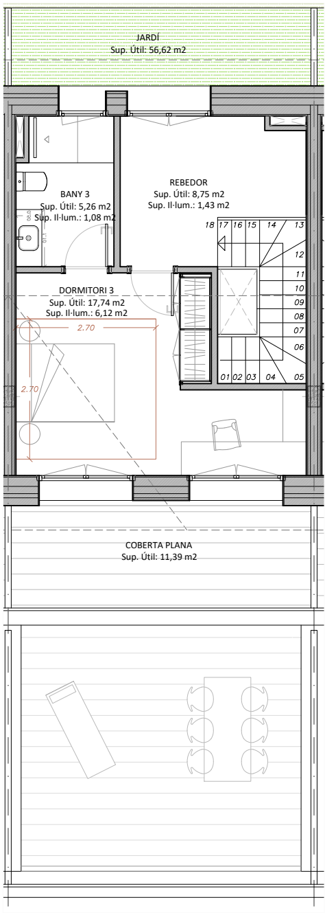
PLANTA SOTACOBERTA
